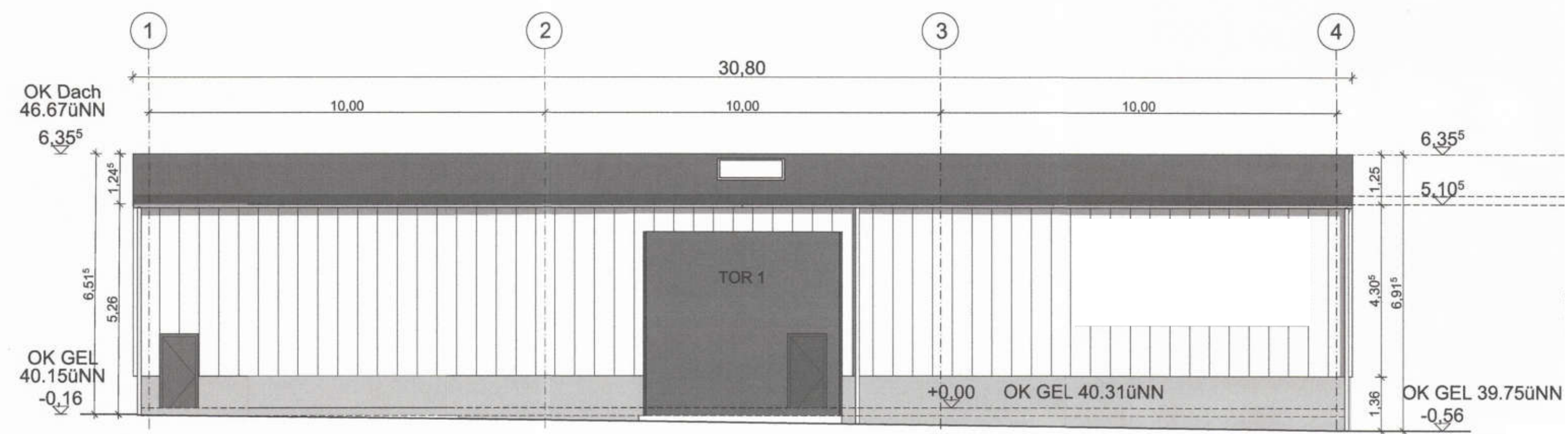
ANSICHT OST
