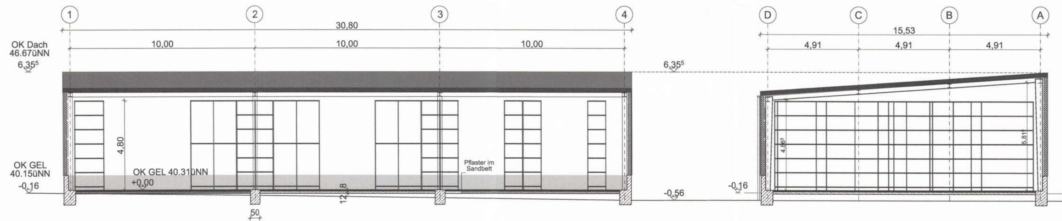
SCHNITT A-A
