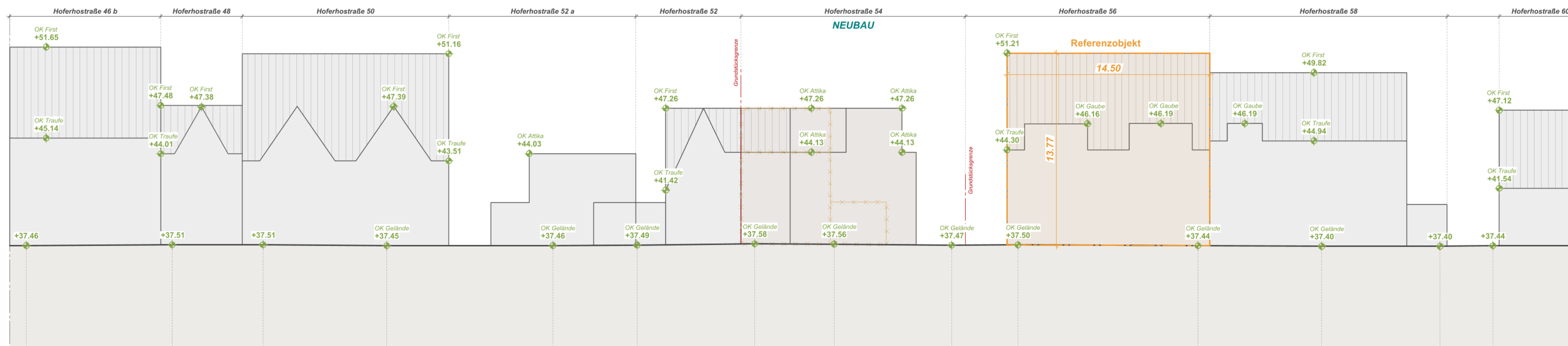
Straßen-Ansicht | M 1: 200
