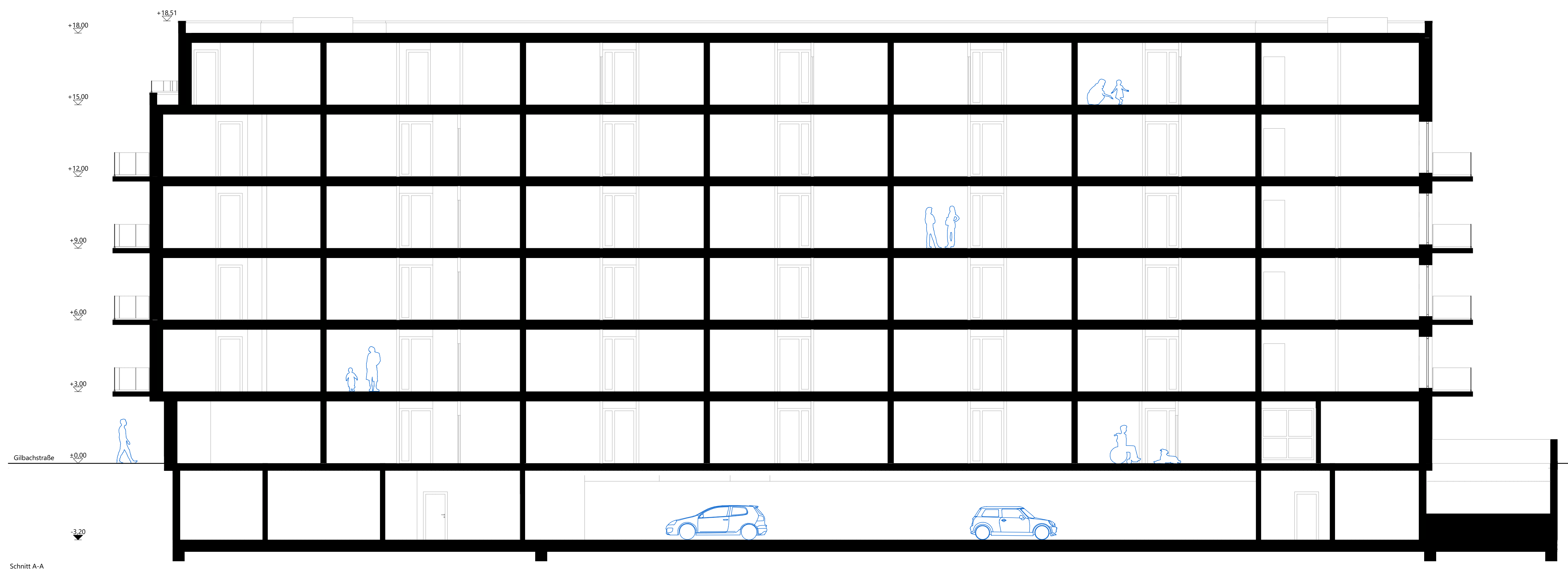
Schnitt A-A
