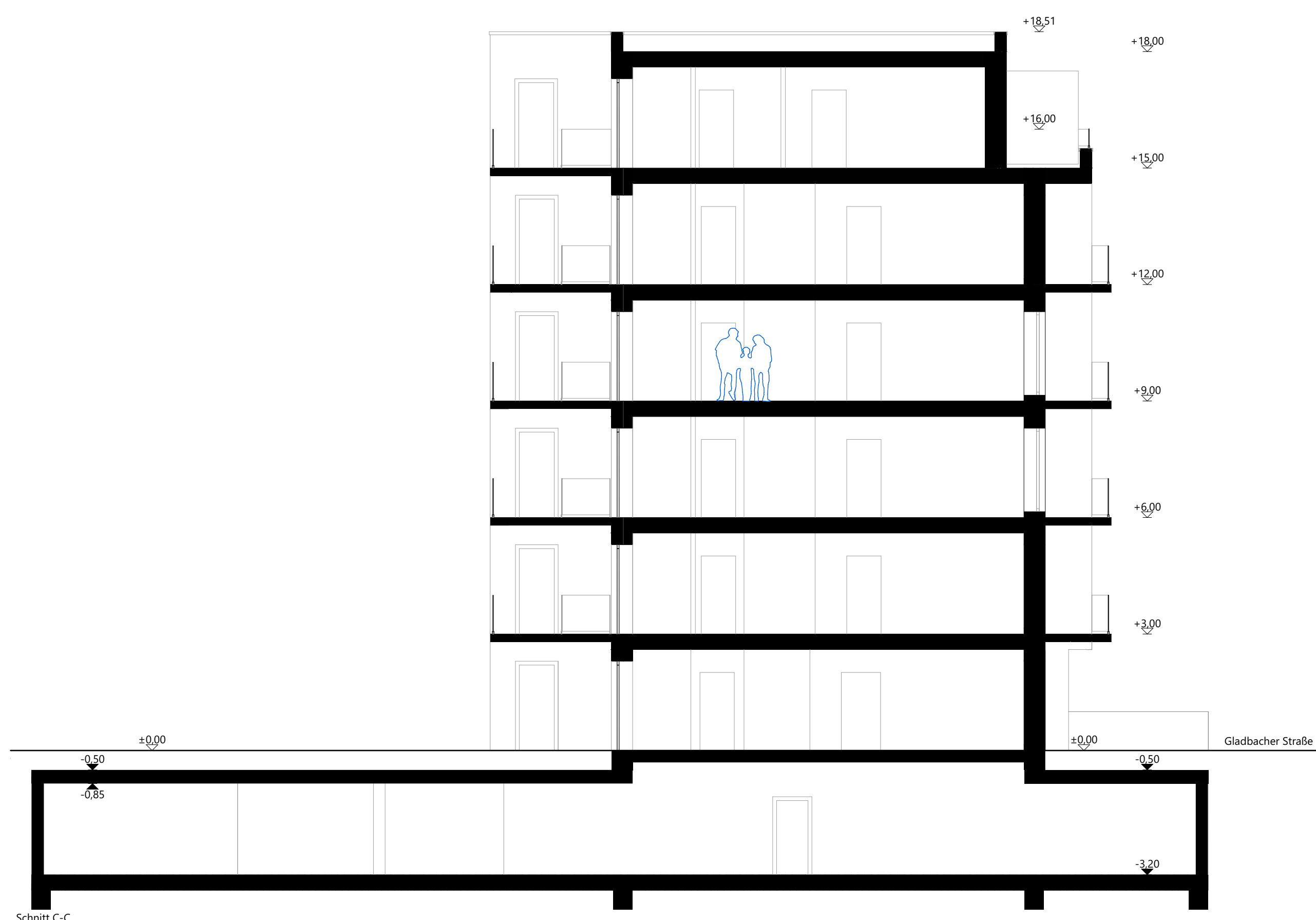
Schnitt C-C
