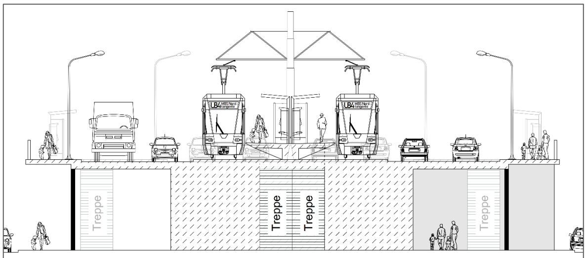
Abbildung 19: Querschnitt Mittellage an der Haltestelle „Theodor-Heuss-Brücke)
