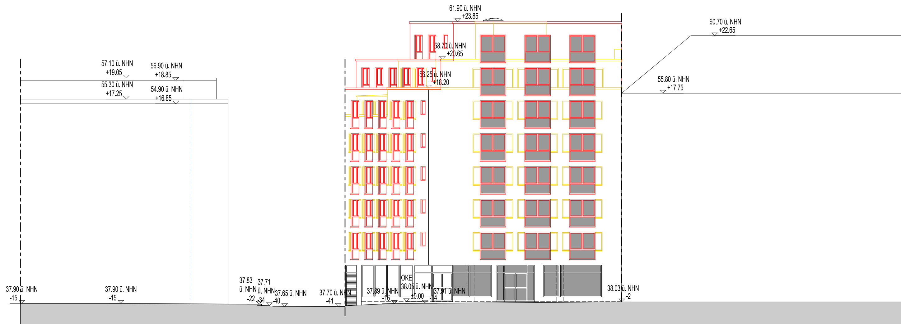
Straßenabwicklung von Karl-Rudolf-Straße
