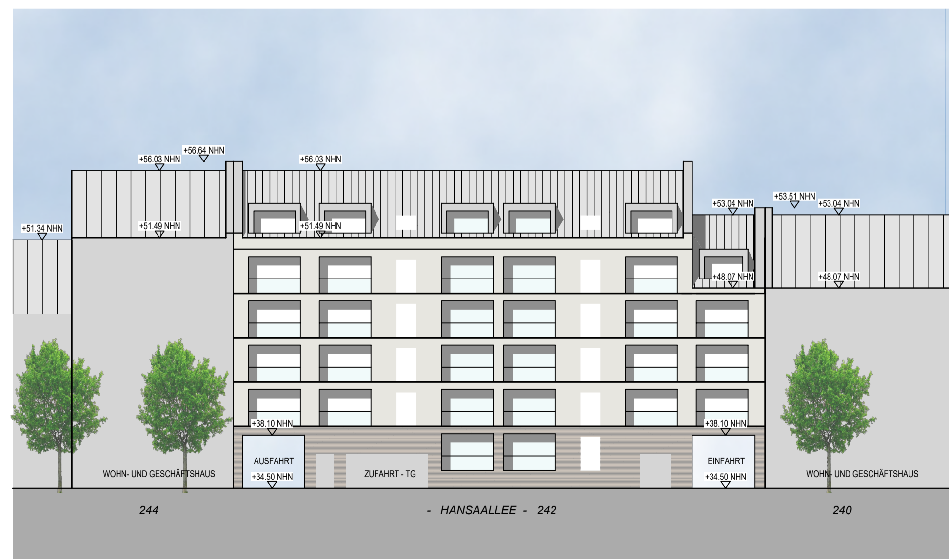
SÜDWESTANSICHT - GEBÄUDE 1
