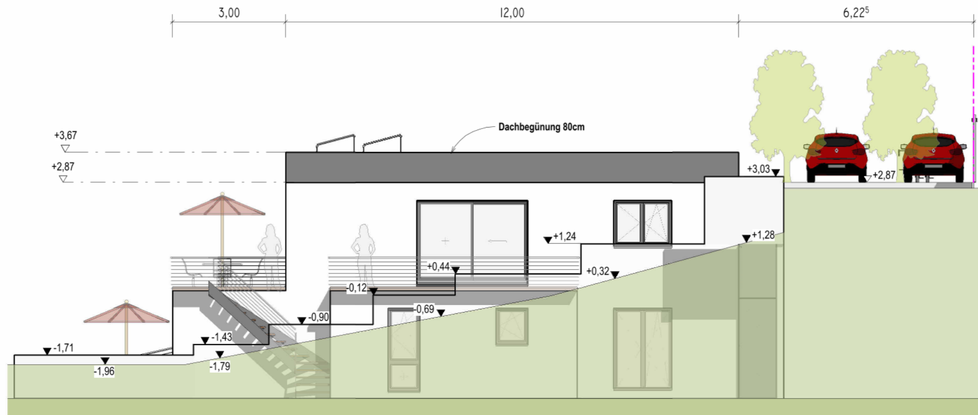
Ansicht Ost
