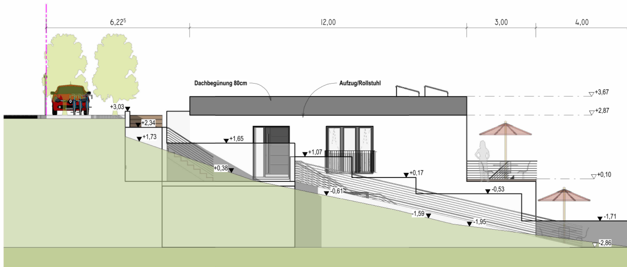
Ansicht West
