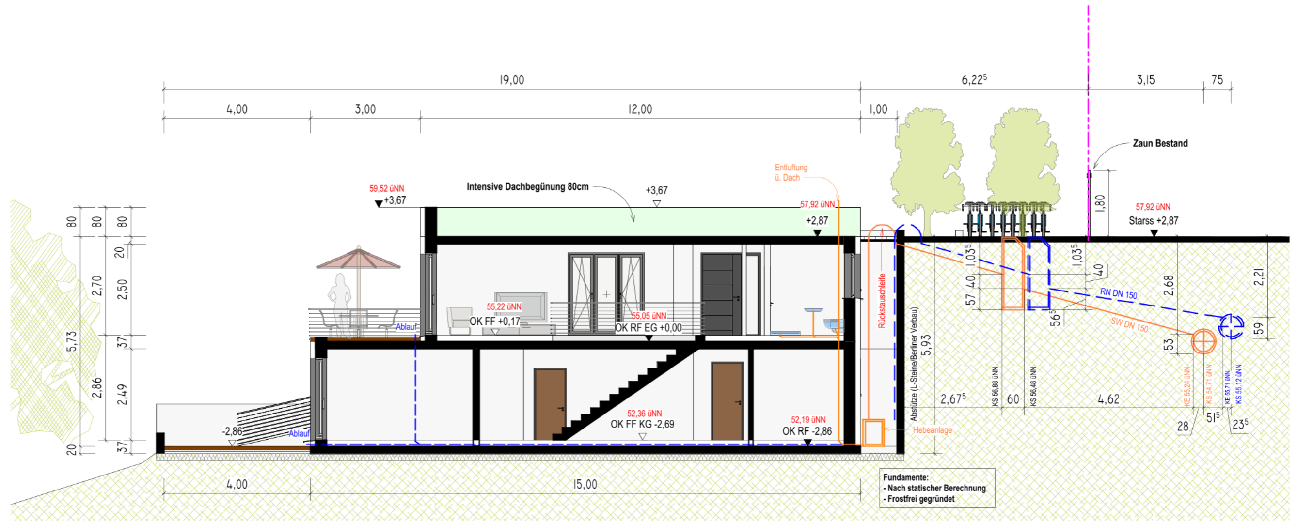
Ansicht A-A
