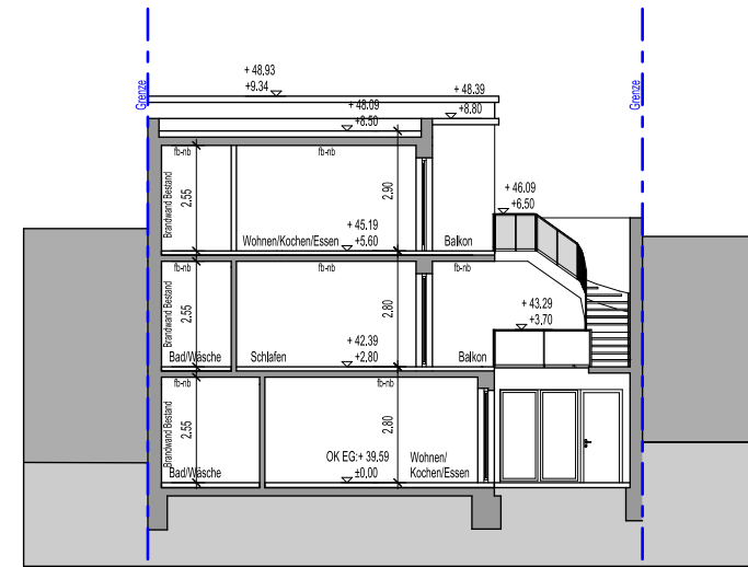
Schnitt B-B
