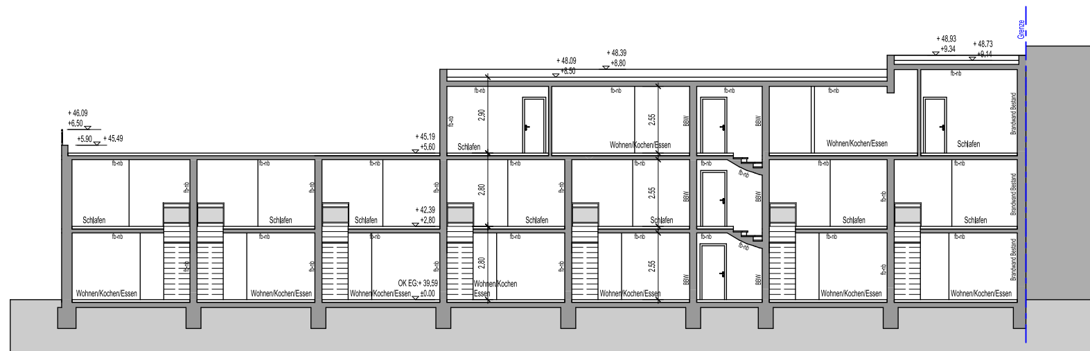
Schnitt C-C
