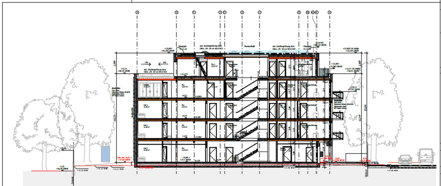
Schnitt AA
