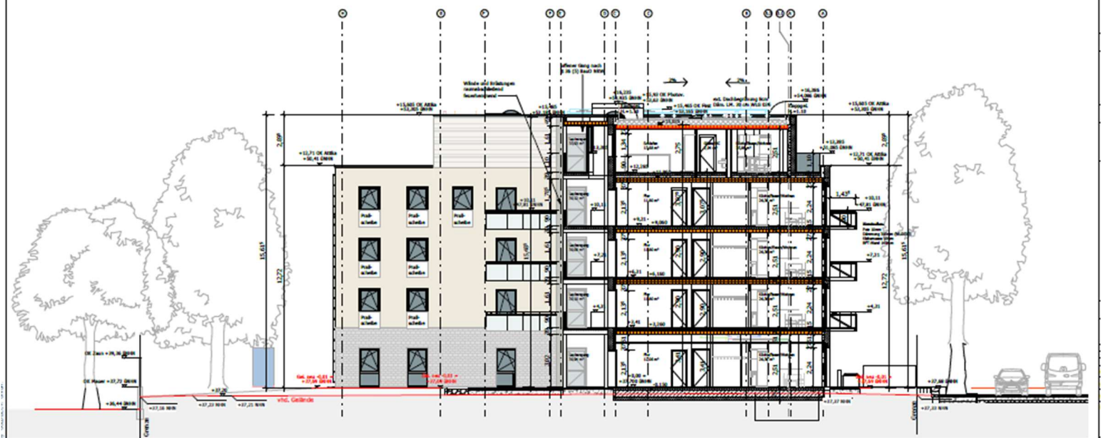
Schnitt BB
