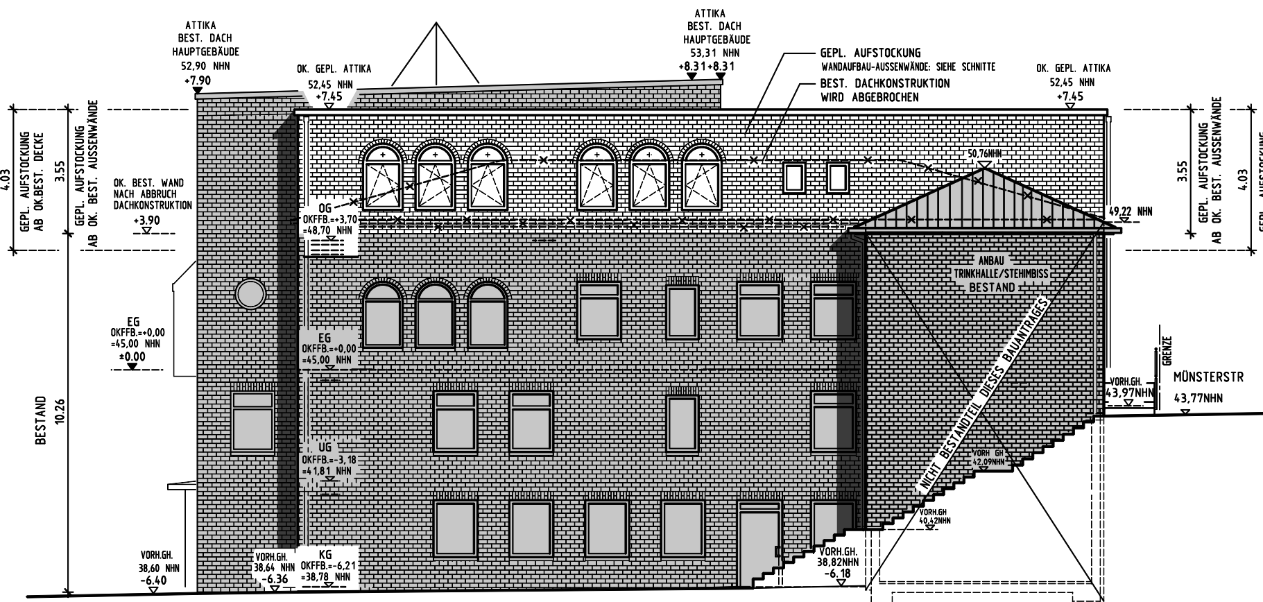
ANSICHT NORD-OST M.1:150
