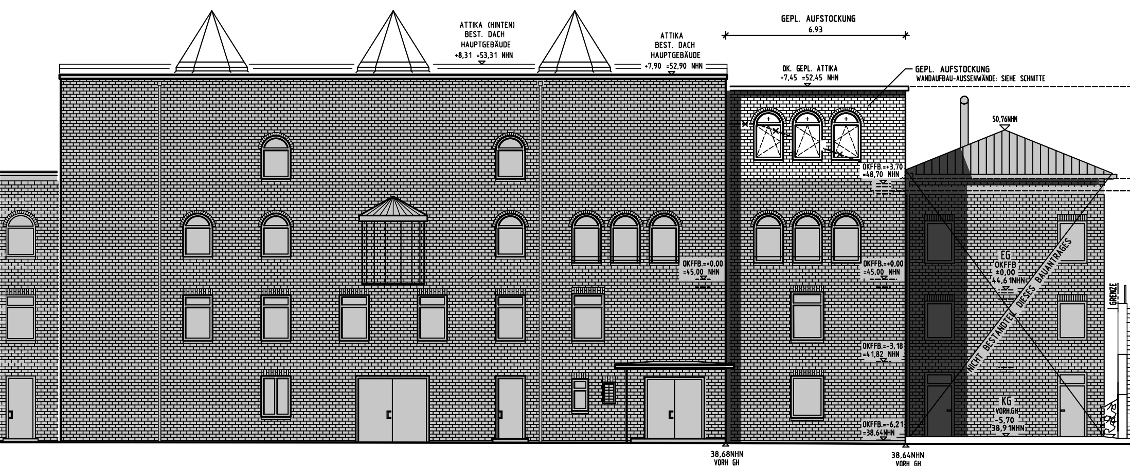
ANSICHT SÜD-OST M.1:150
