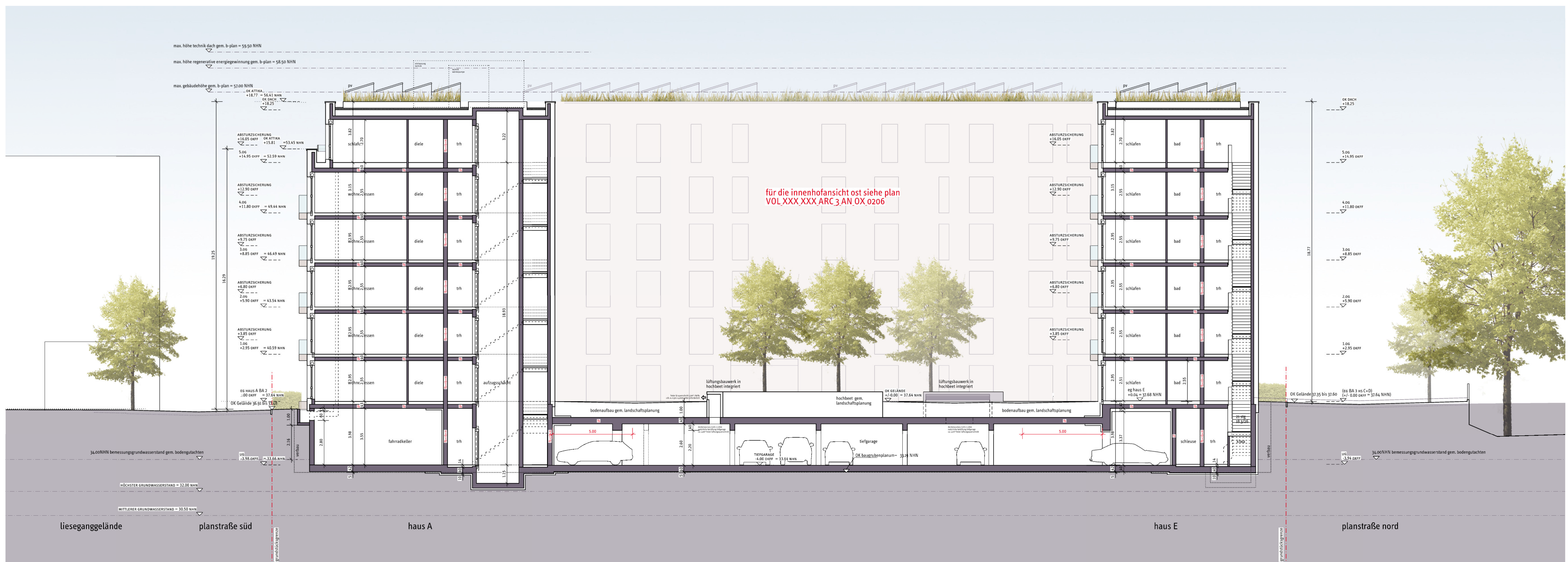
schnitt B-B
