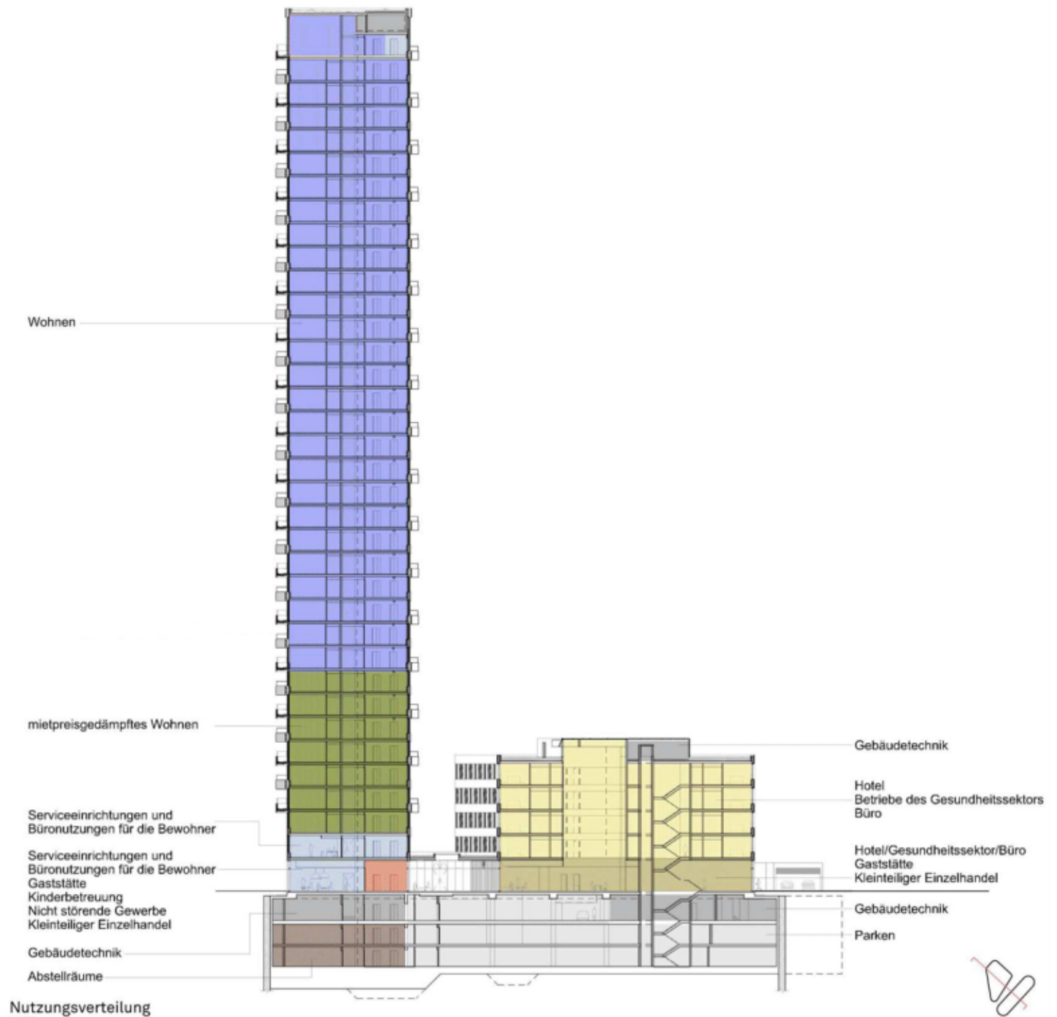
Schnitt - Mietpreisgedämpftes Wohnen - Neustand Nutzungsverteilung
