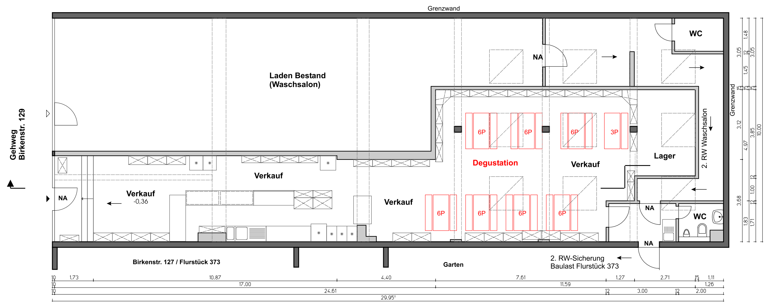
Grundriss/Schnitt M 1:100
