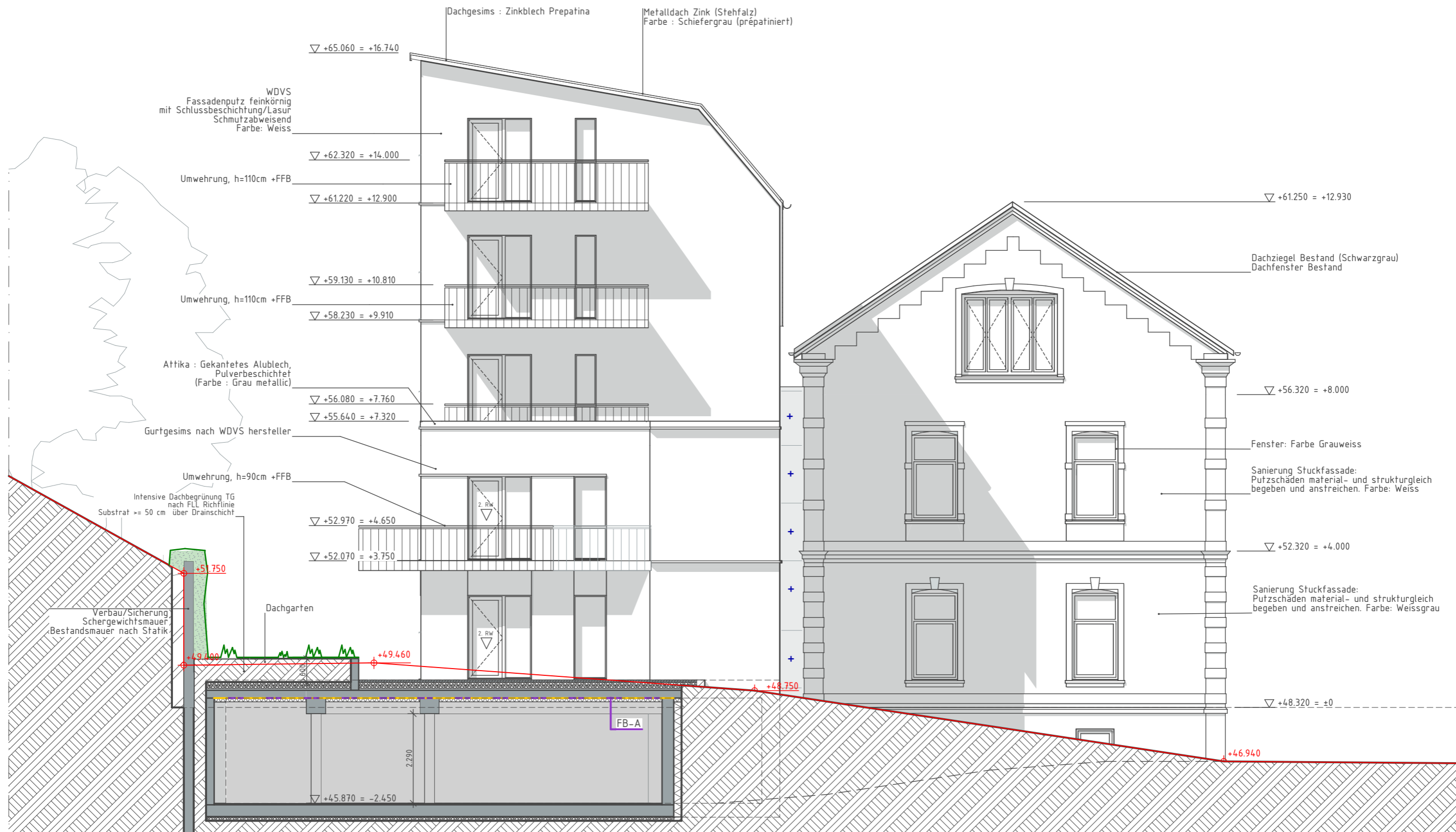
Ansicht Links
