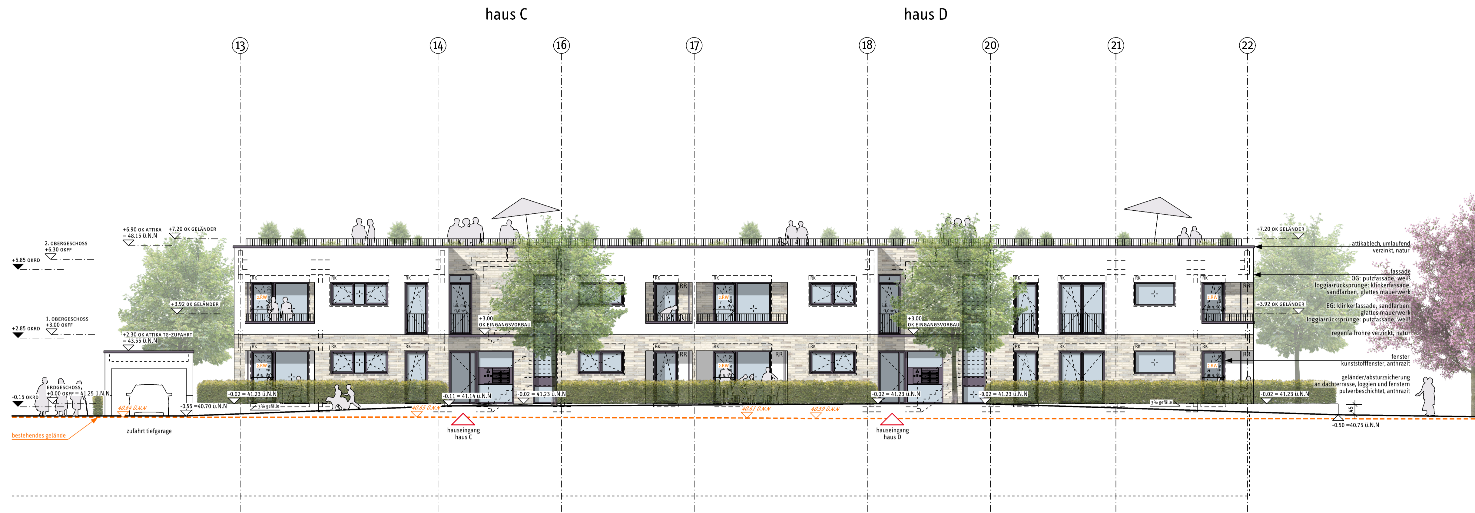
haus C,D | ansicht süden m 1:100
