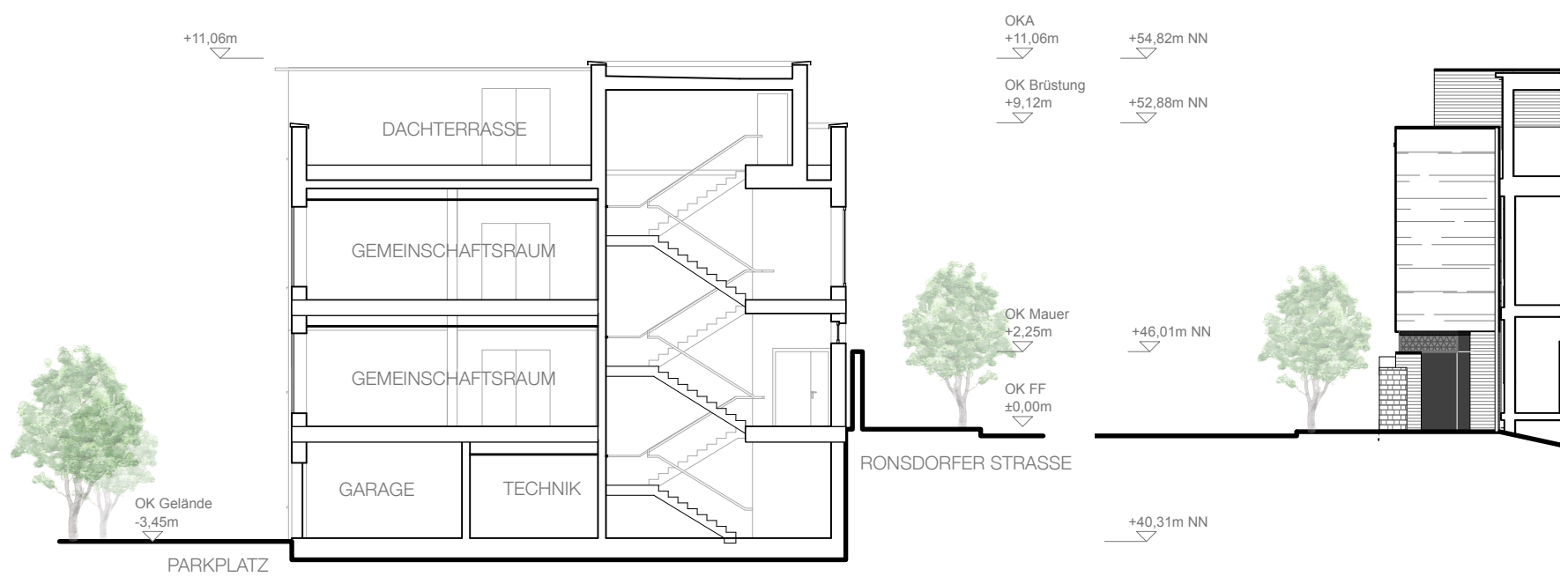
Schnitt AA
