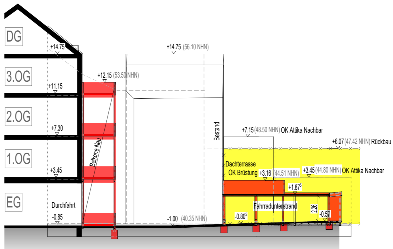
Schnitt C - C
