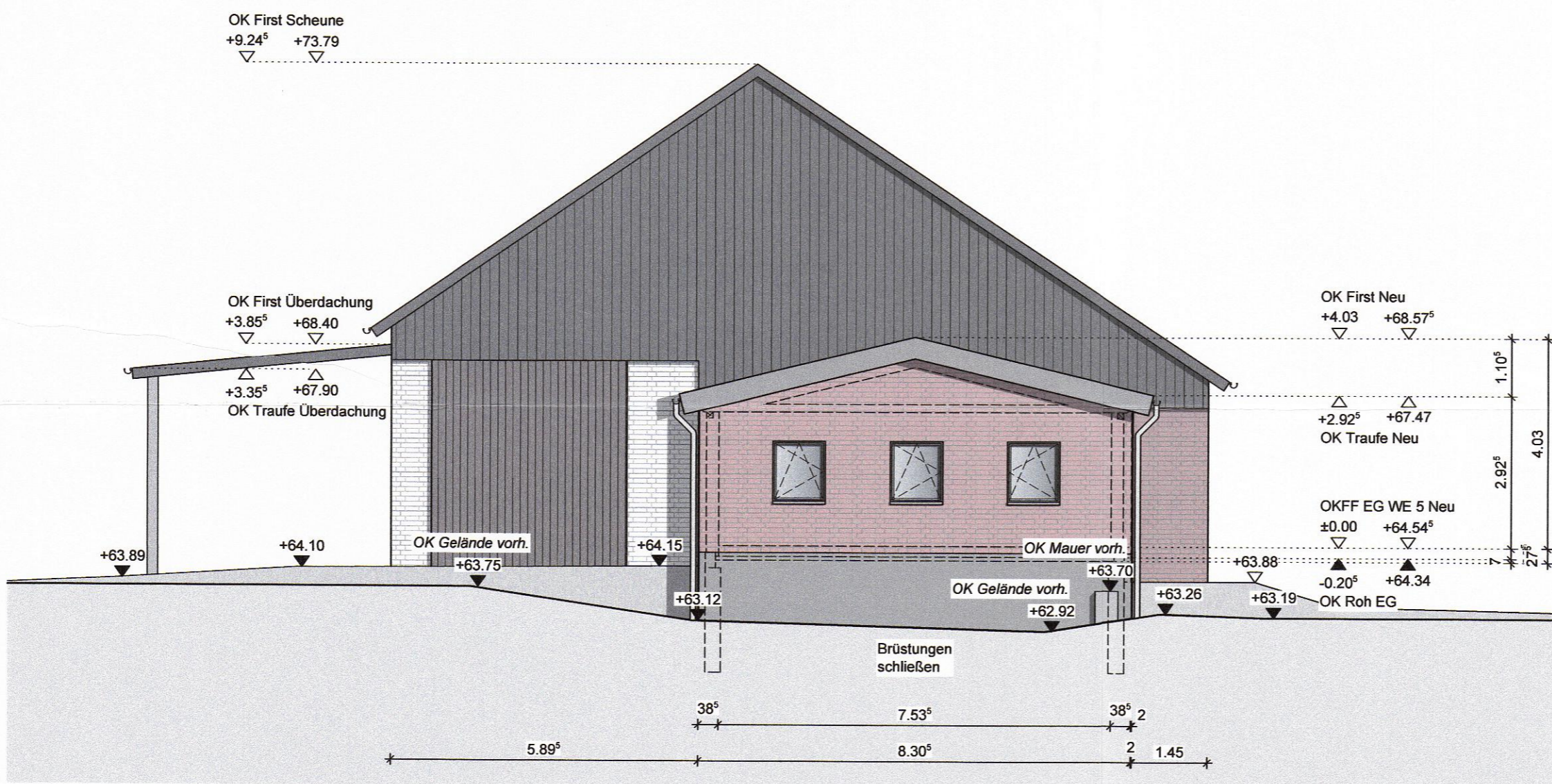
ANSICHT SÜD (RECHTER GIEBEL)
