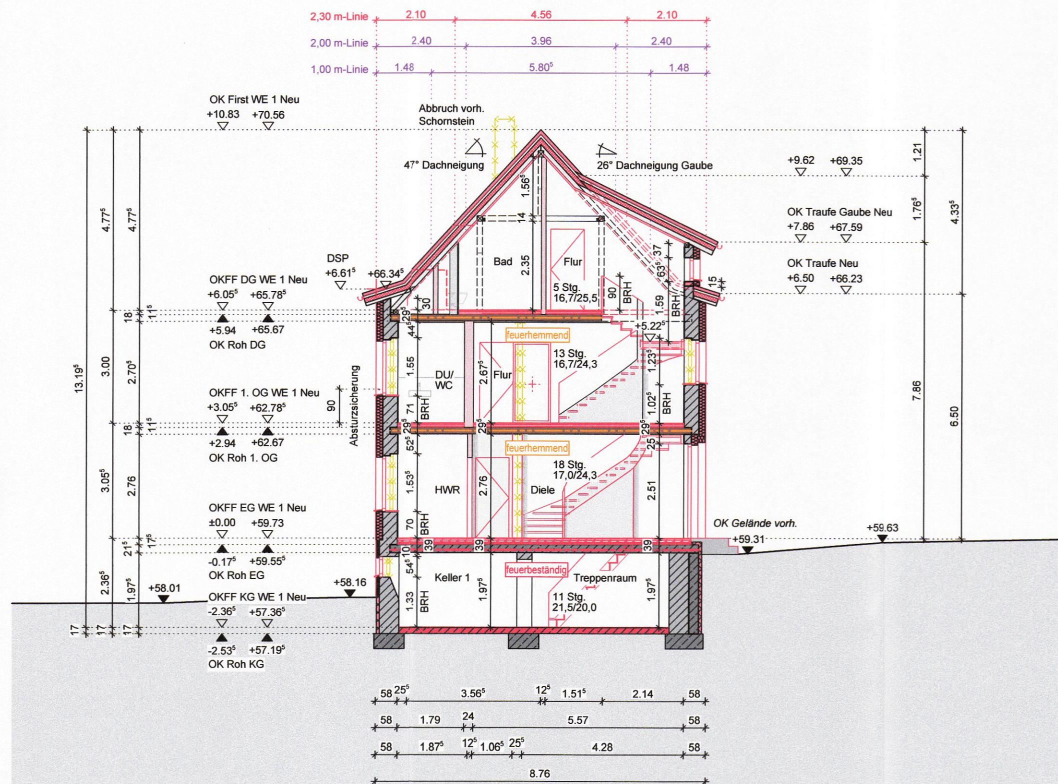
SCHNITT A-A
