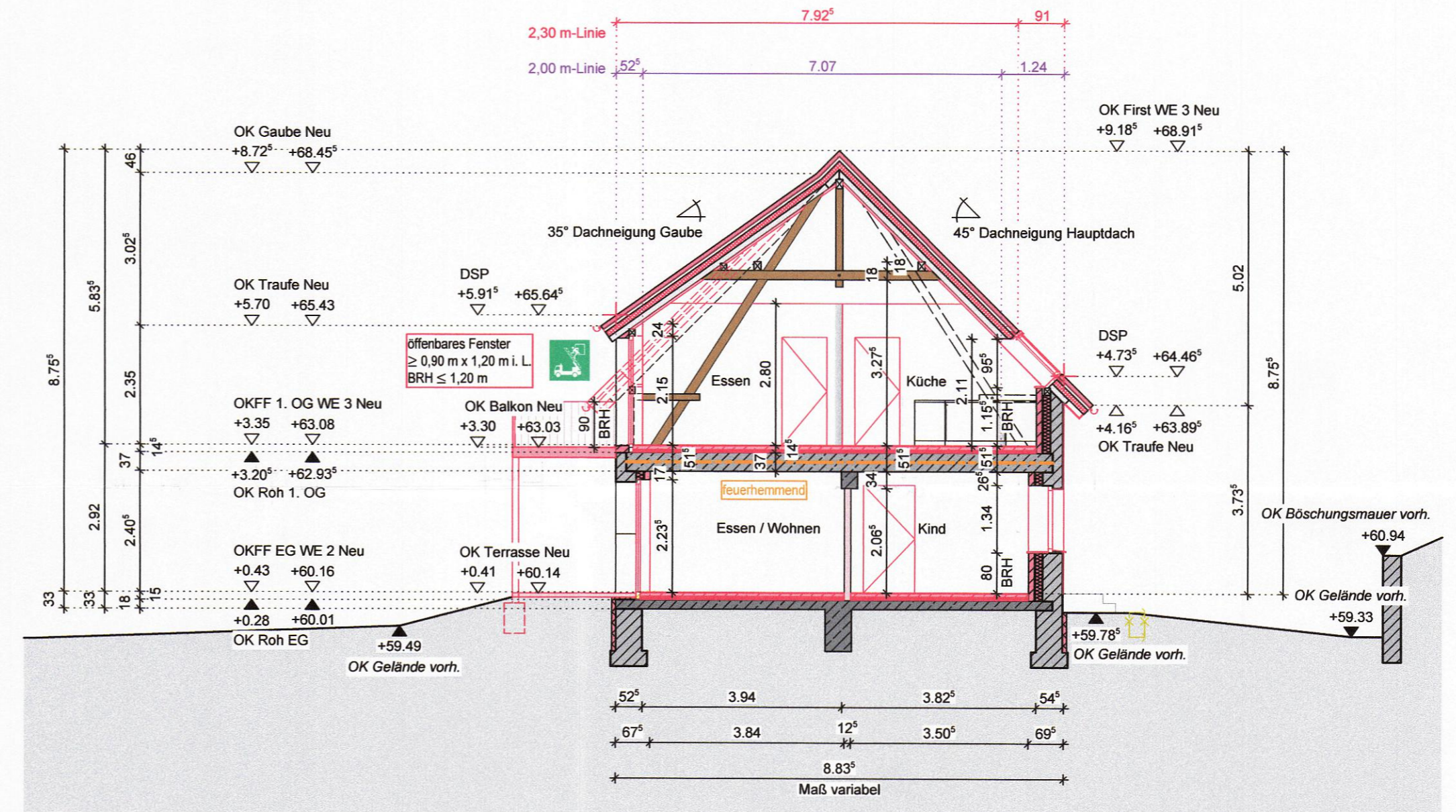
SCHNITT B-B
