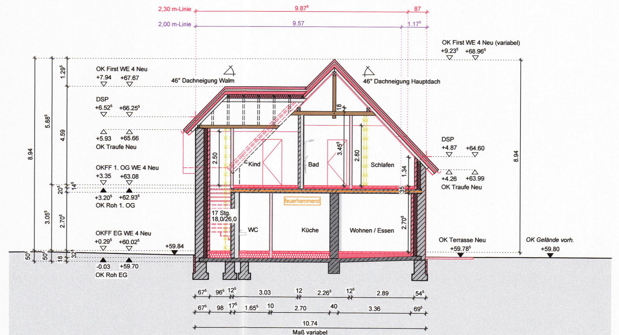
SCHNITT C-C
