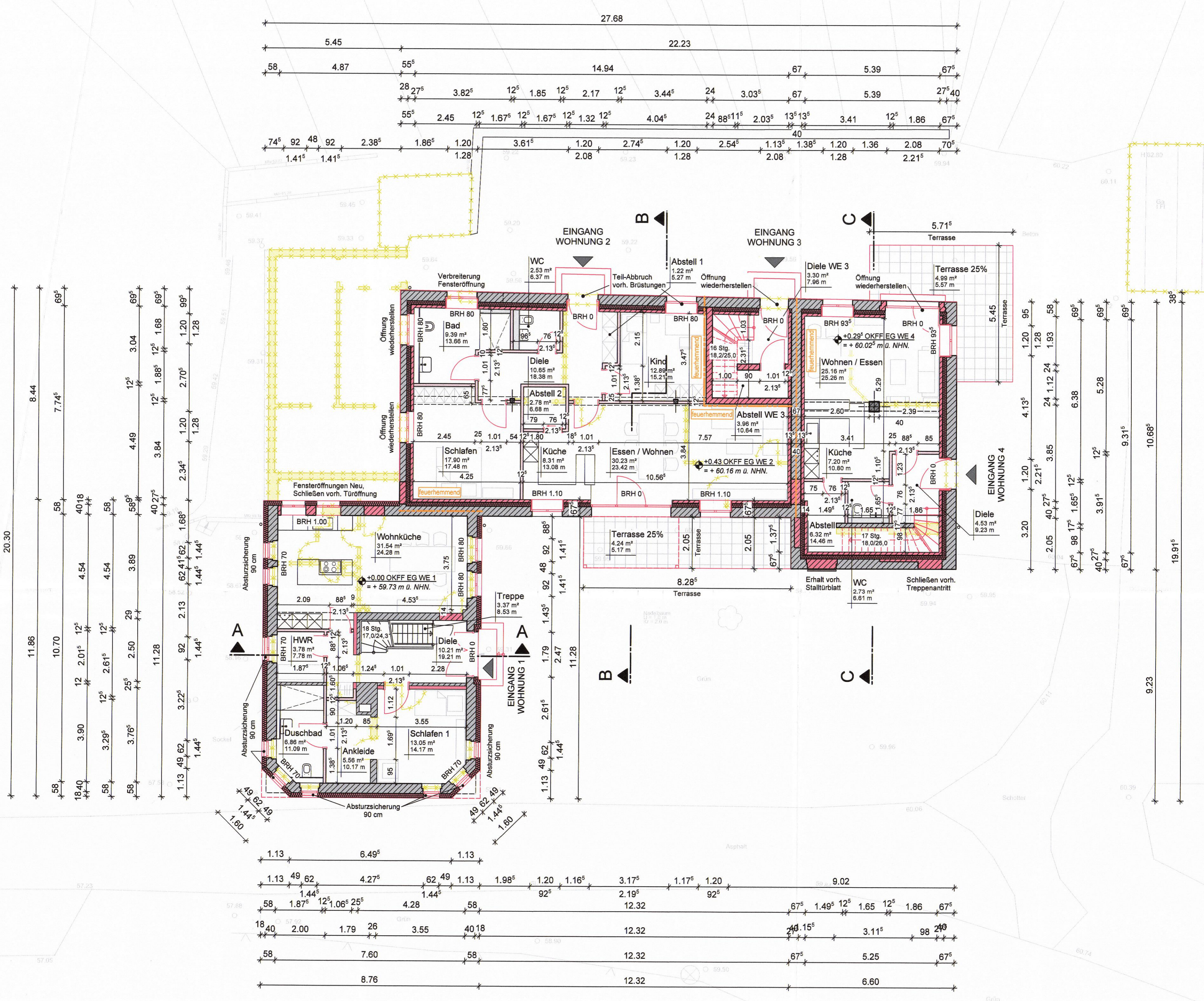
GRUNDRISS ERDGESCHOSS
