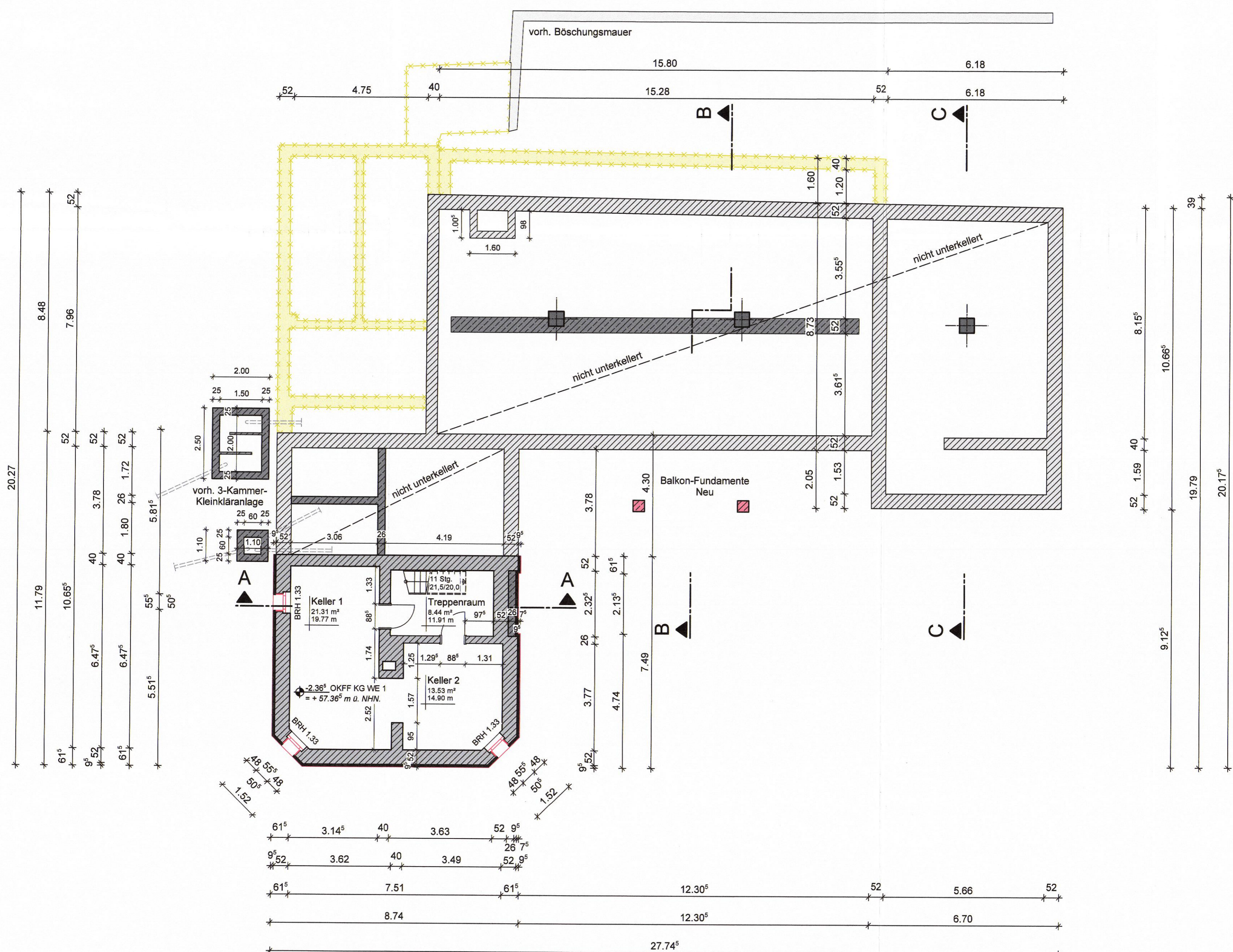
GRUNDRISS KELLERGESCHOSS
