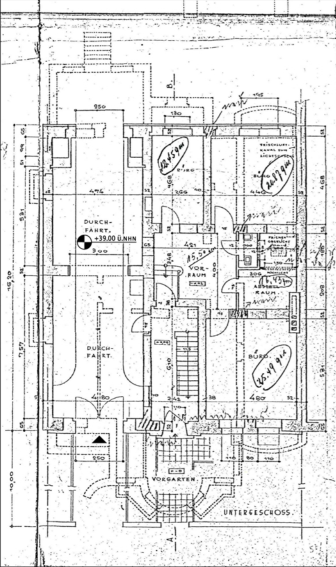
grundriss untergeschoss, ebene der durchfahrt
