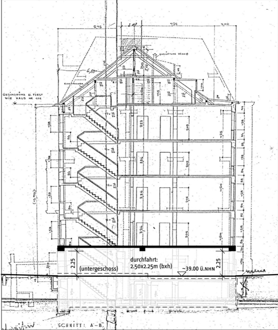
schnitt a-b
