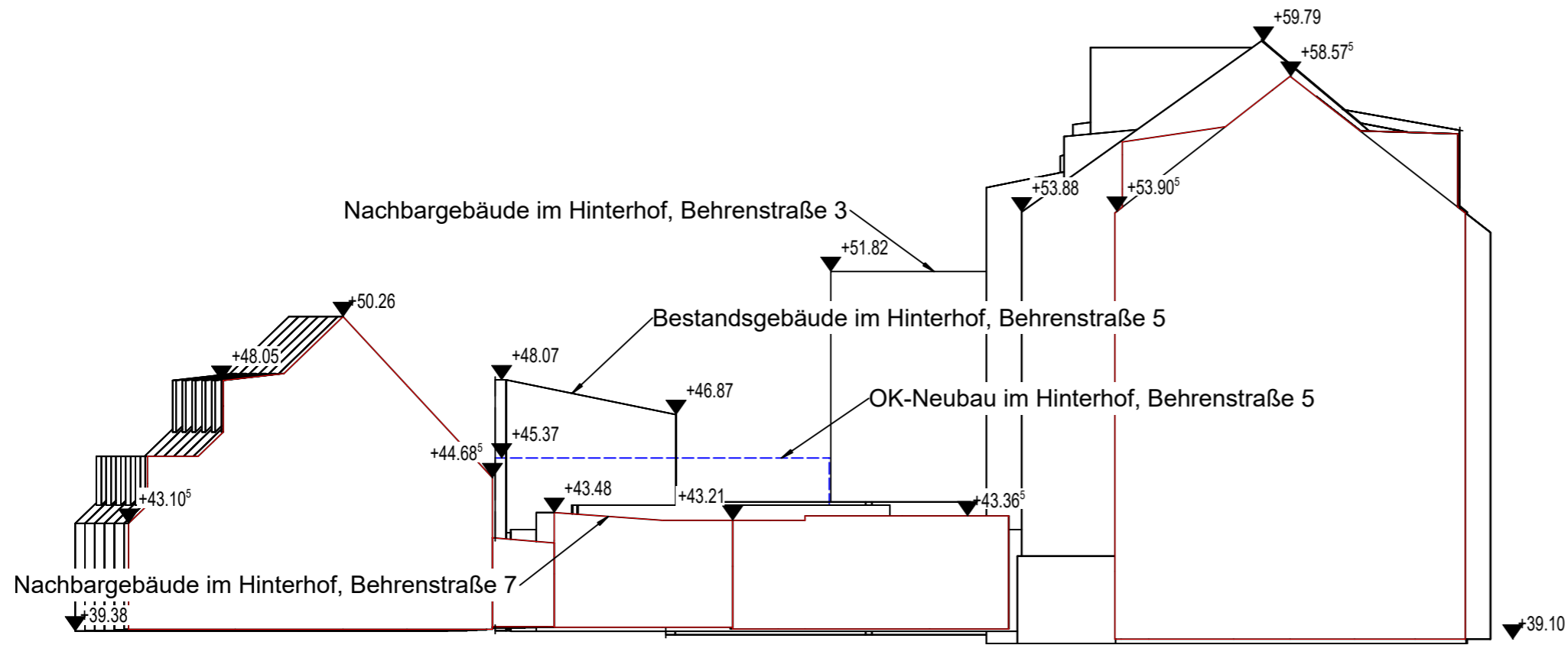
Schnitt B-B aus digitalem Stadtmodell Düsseldorf
