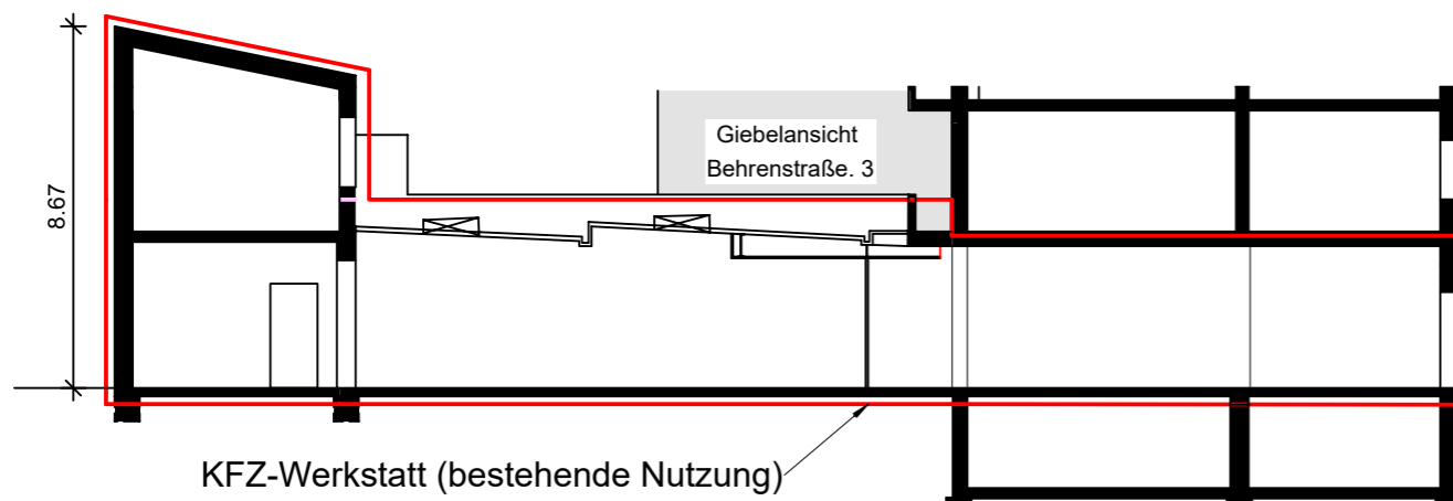
Schnitt Bestand
