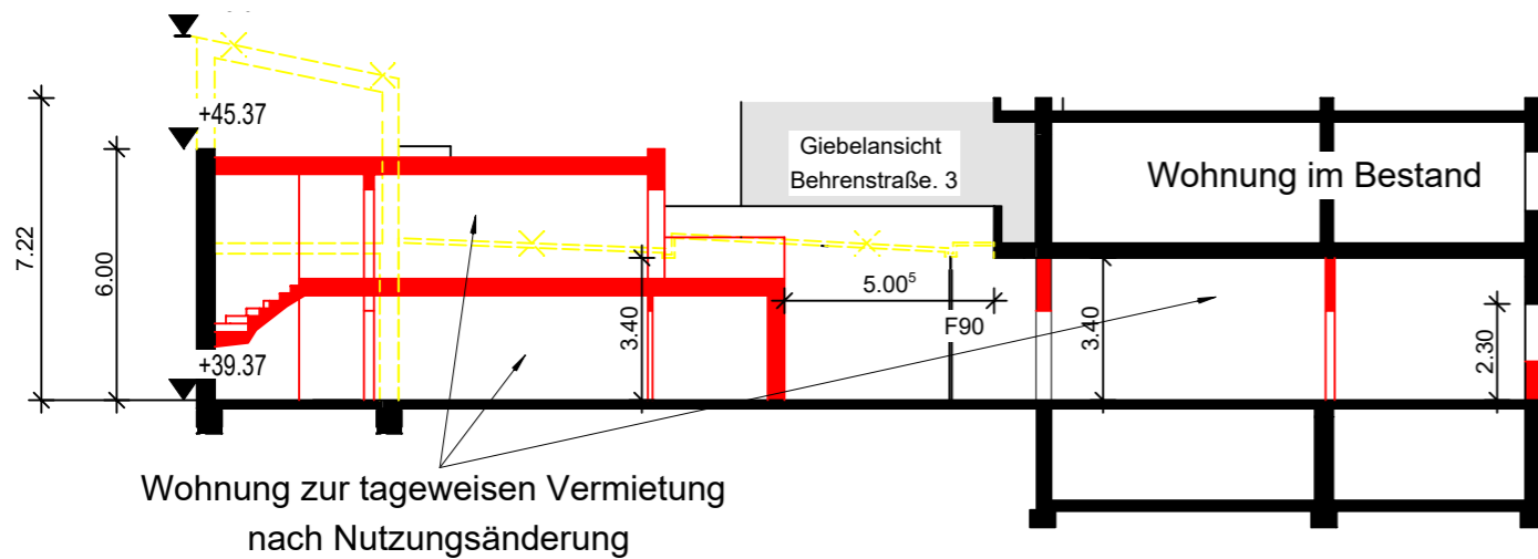
Schnitt nach Umbau
