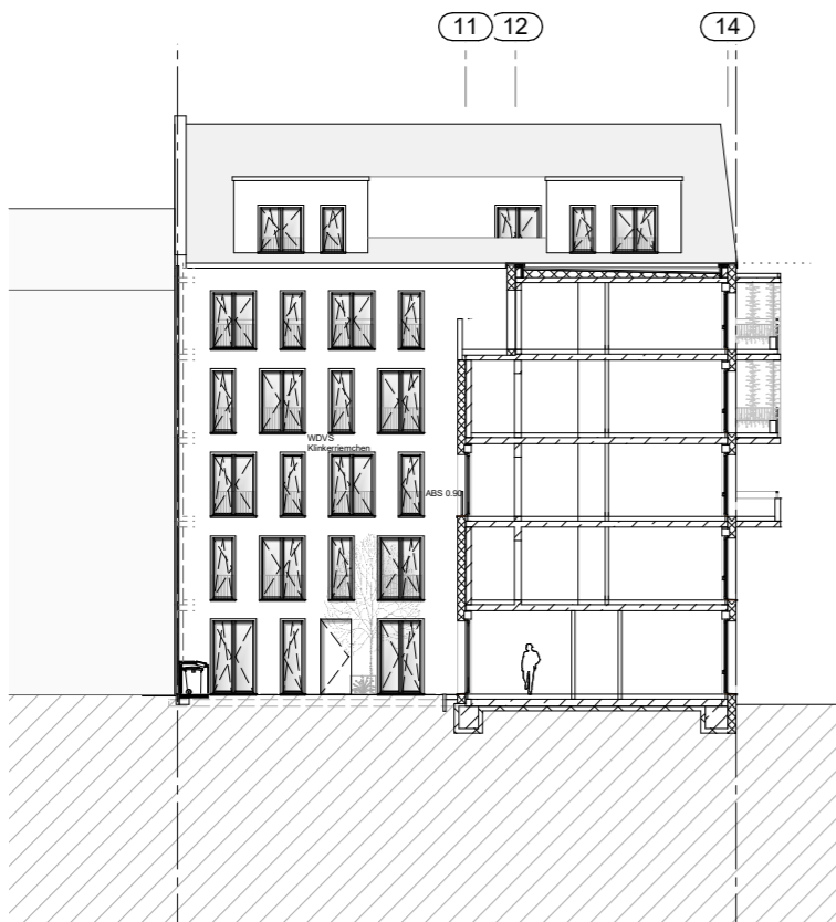
Schnitt AA | Ansicht WEST | Haus 1
