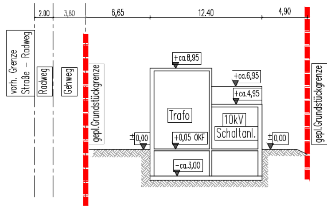
SKIZZE: SYSTEMSCHNITT B-B
