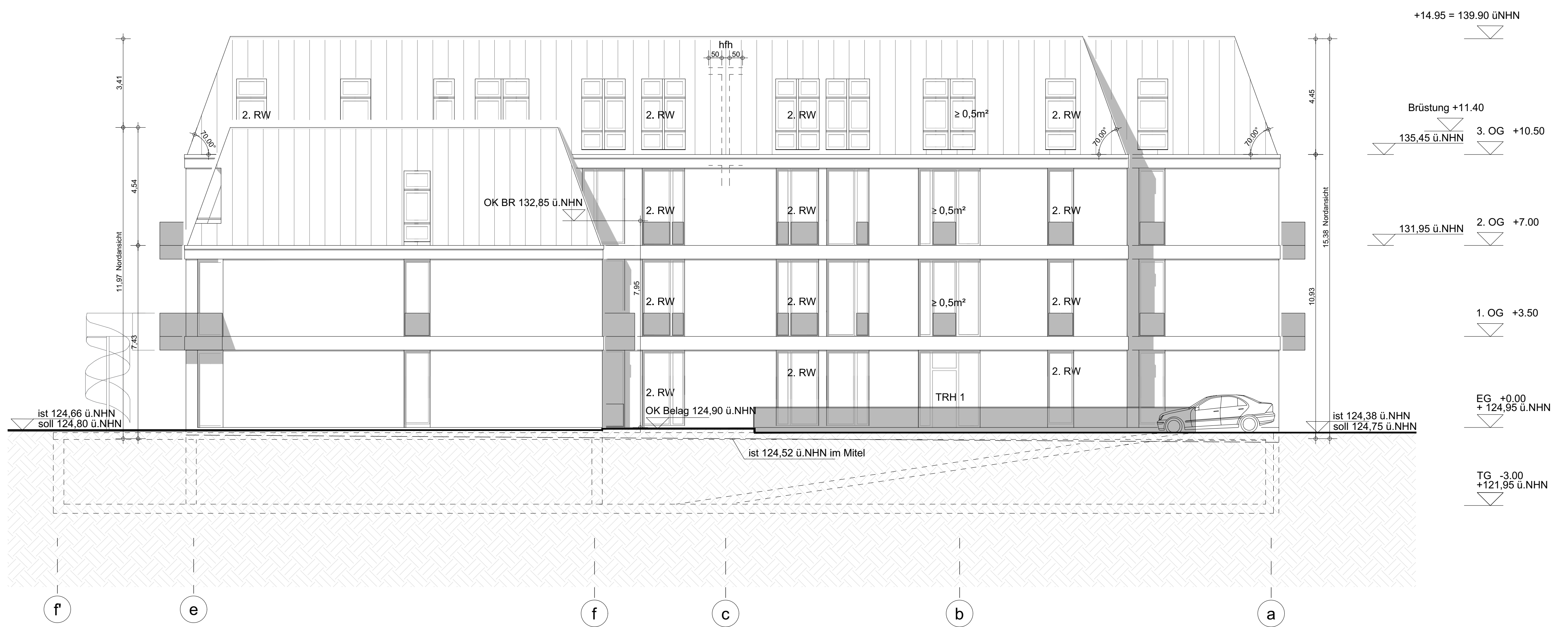
Nordansicht
