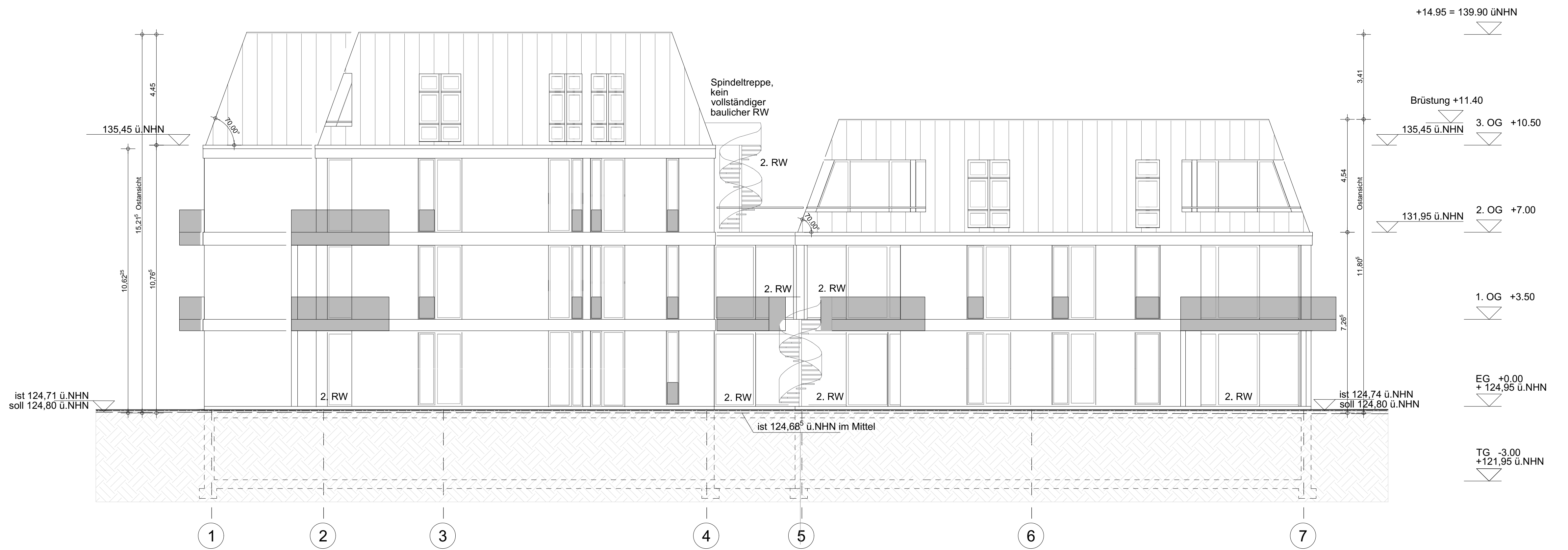
Ostansicht
