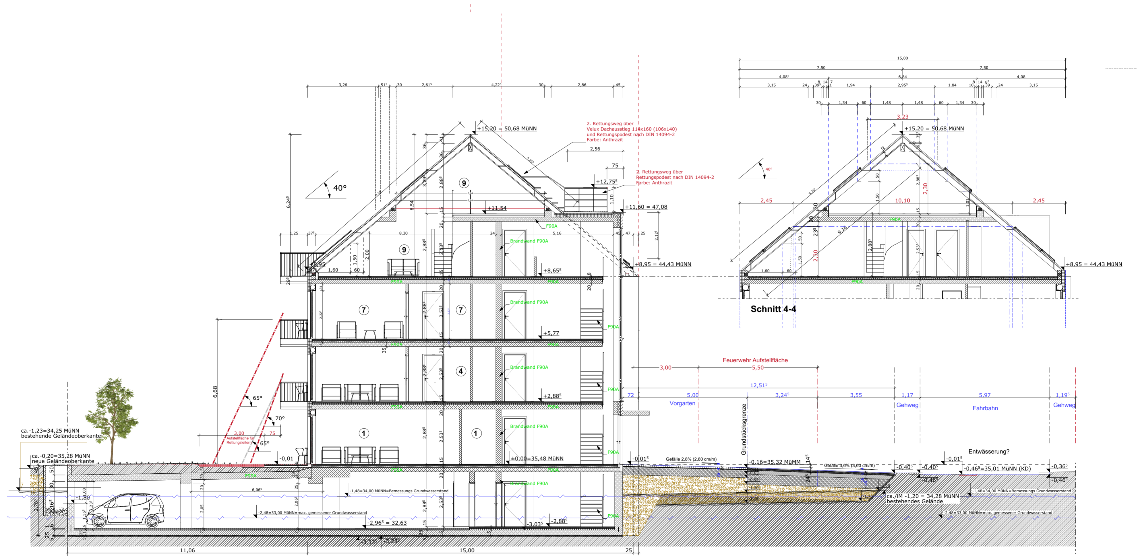
Schnitt 1-1
