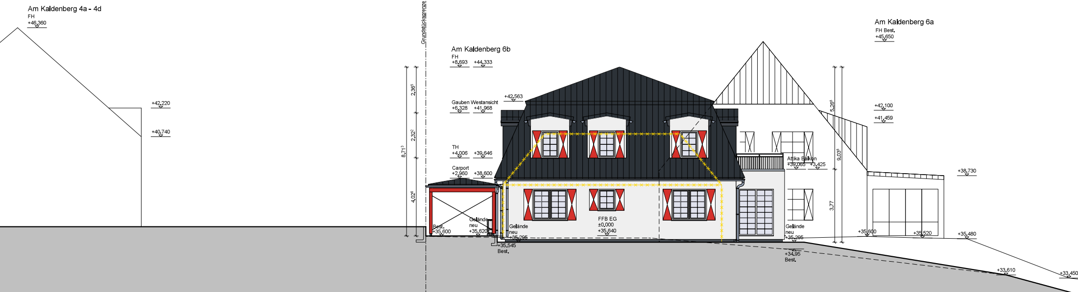
Westansicht M 1:100
