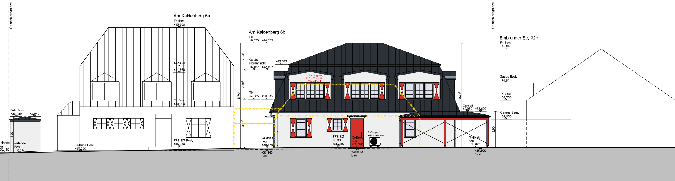
Nordansicht M. 1:100
