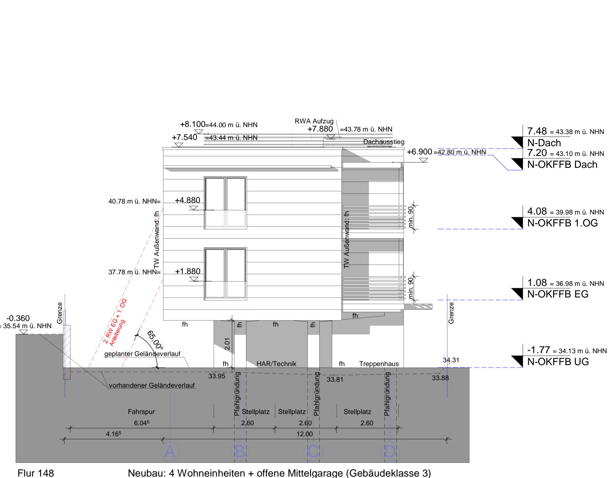
Flur 148 Neubau: 4 Wohneinheiten + offene Mittelgarage (Gebäudeklasse 3)
