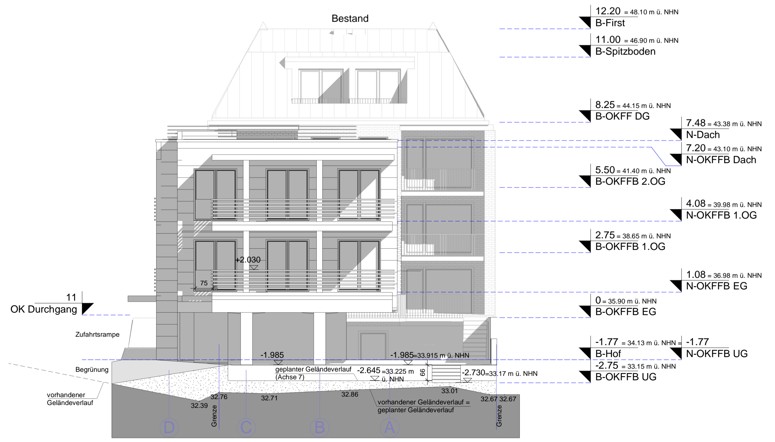
Neubau: 4 Wohneinheiten + offene Mittelgarage (Gebäudeklasse 3)
