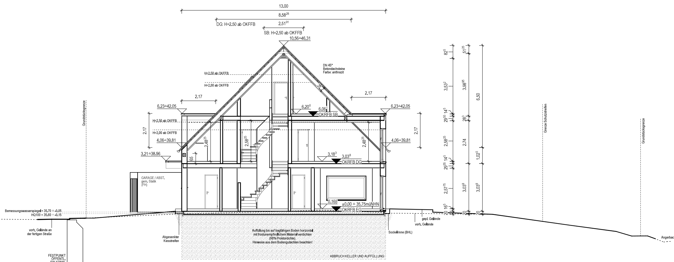
SCHNITT quer
