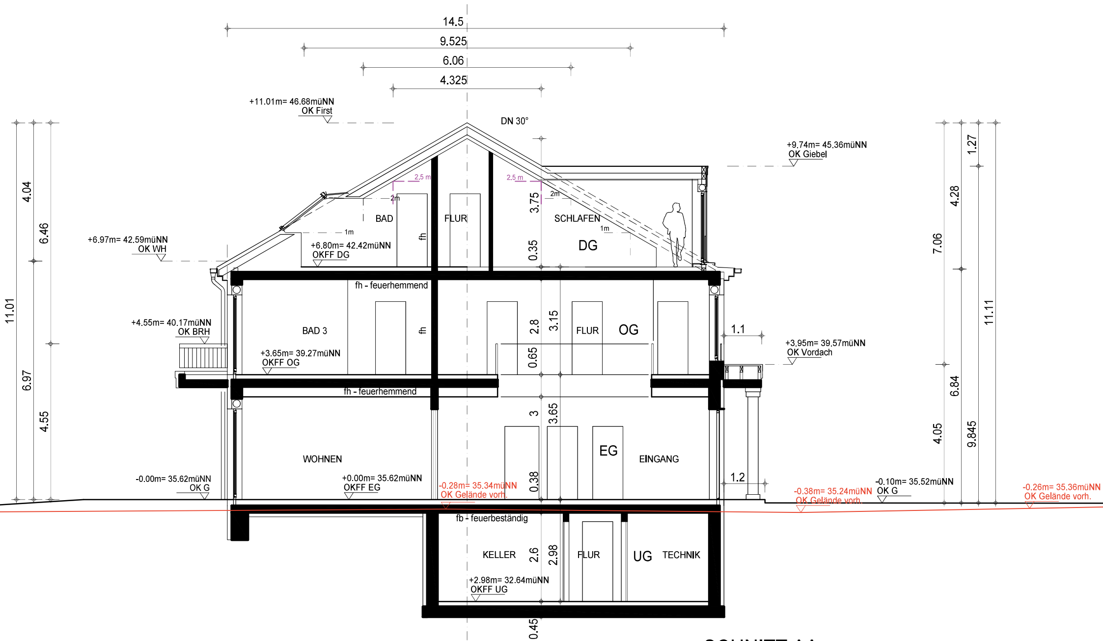
SCHNITT AA DH-H B
