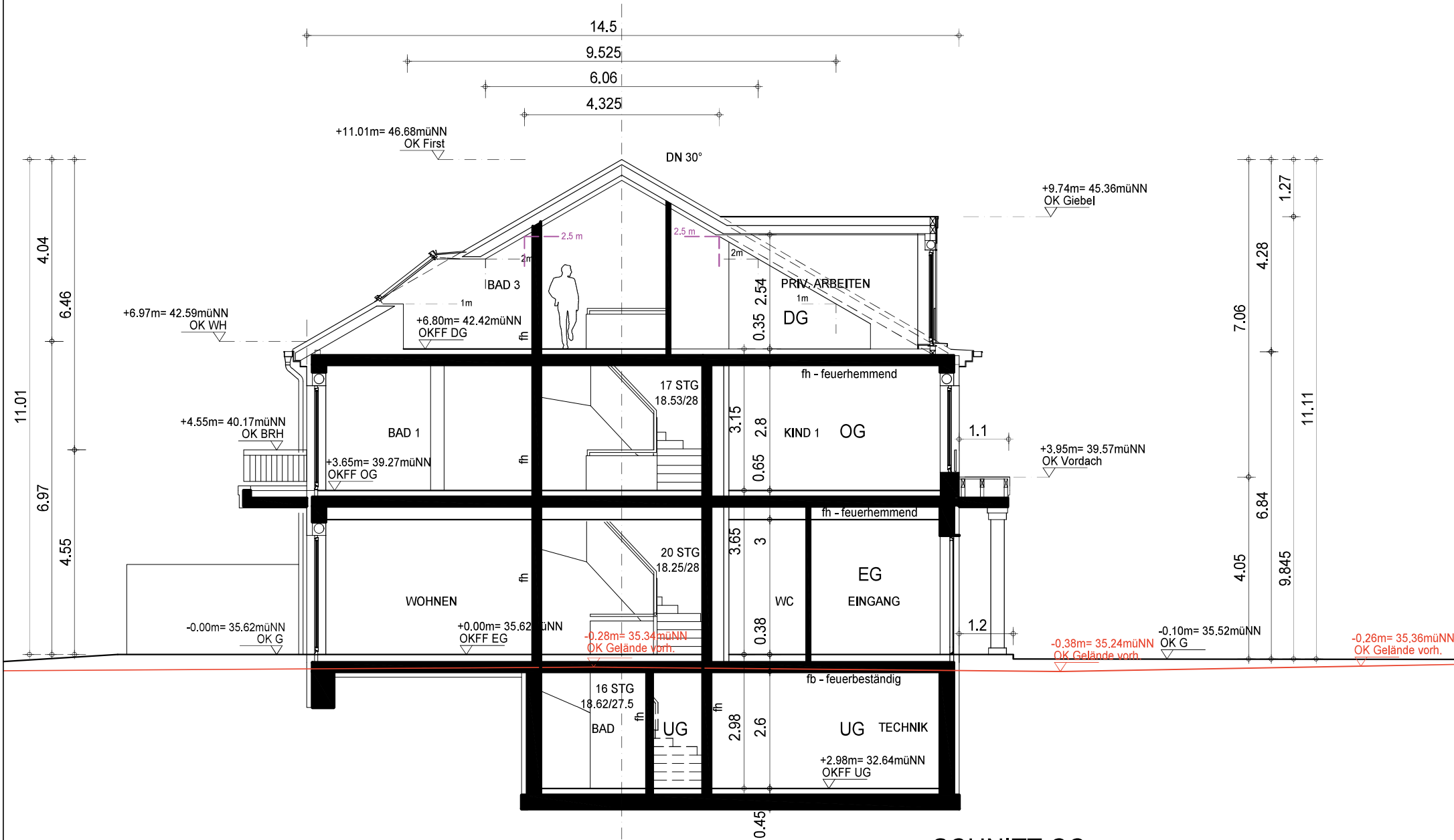
SCHNITT CC DH-H A
