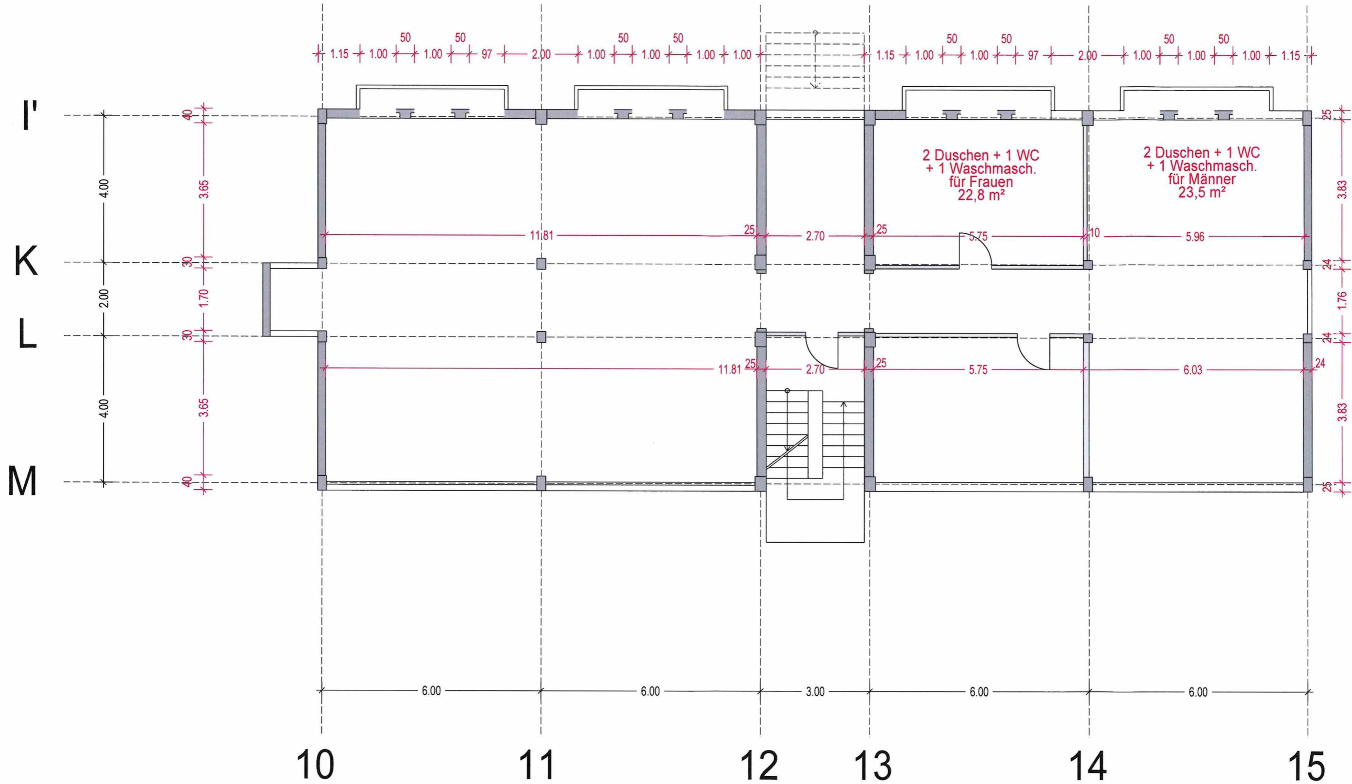
Untergeschoss 1:100
