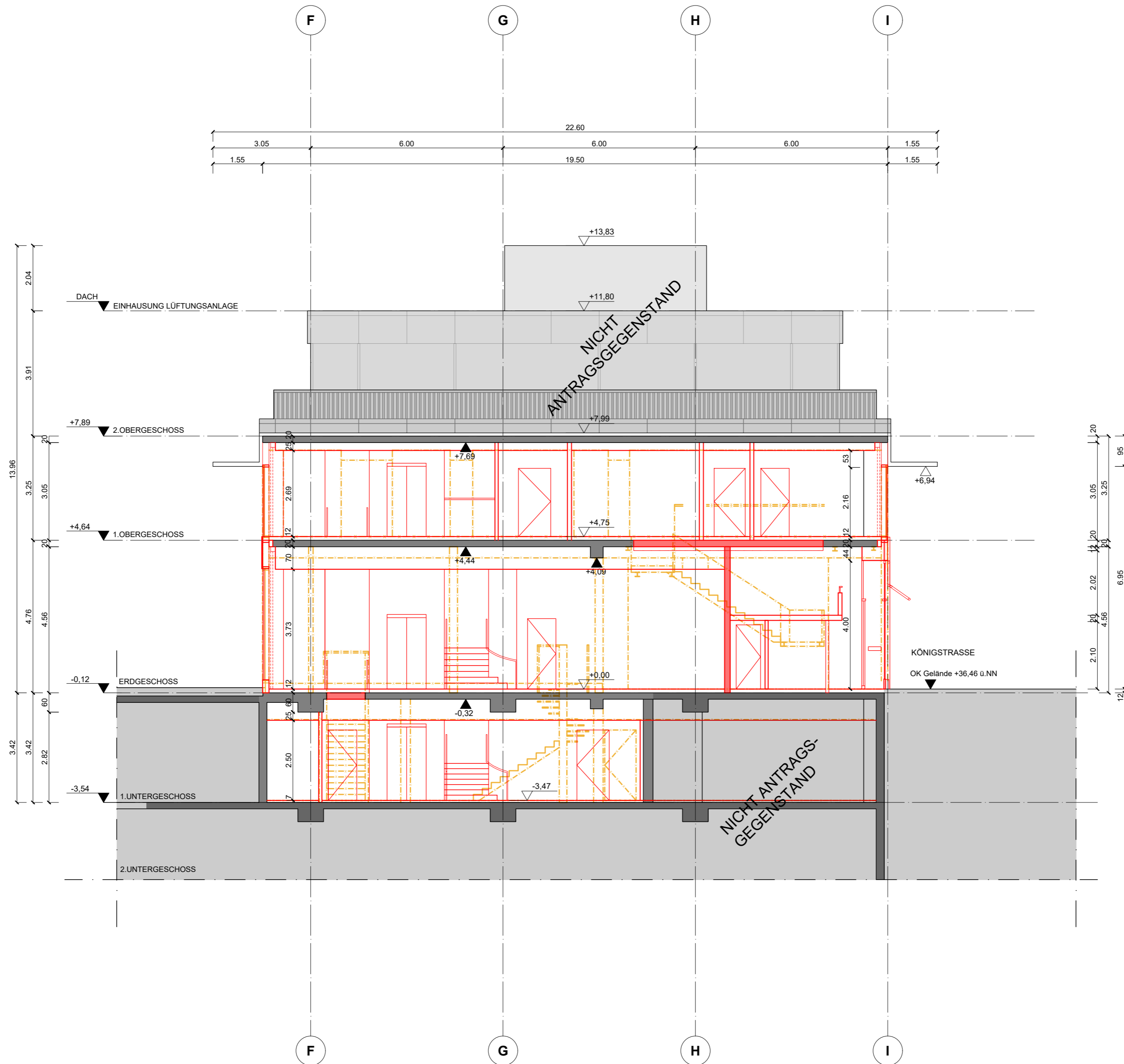
Schnitt A-A'
