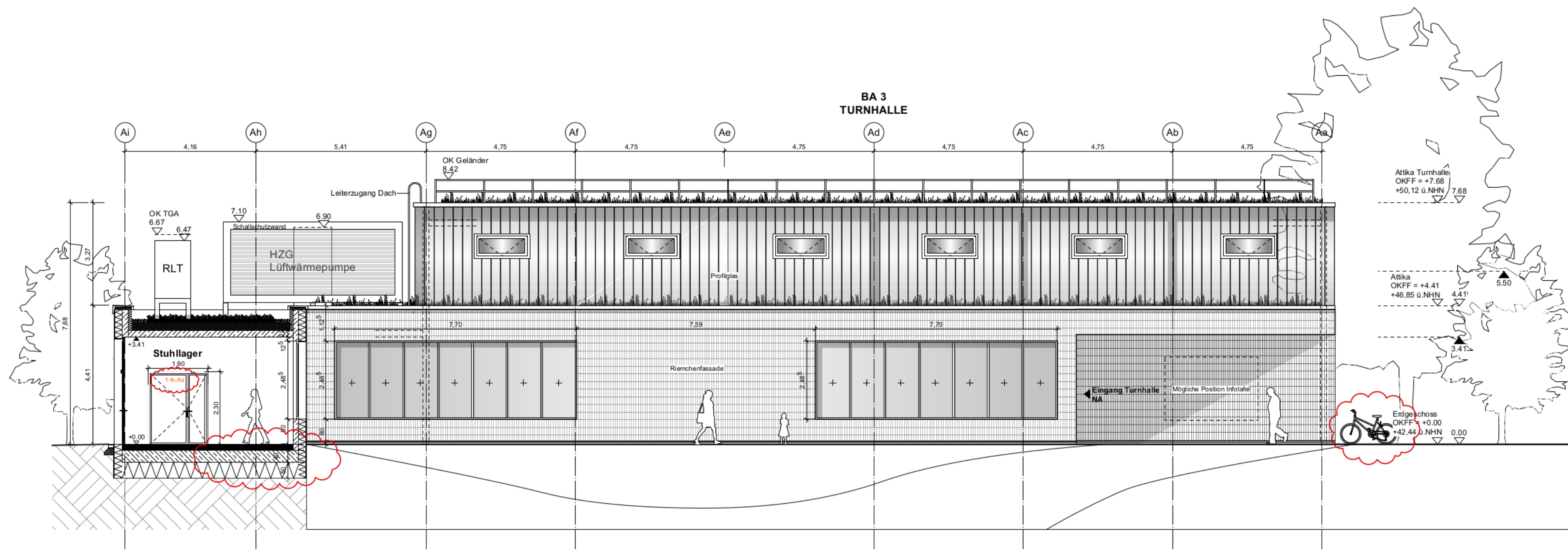
Ansicht West Turnhalle
